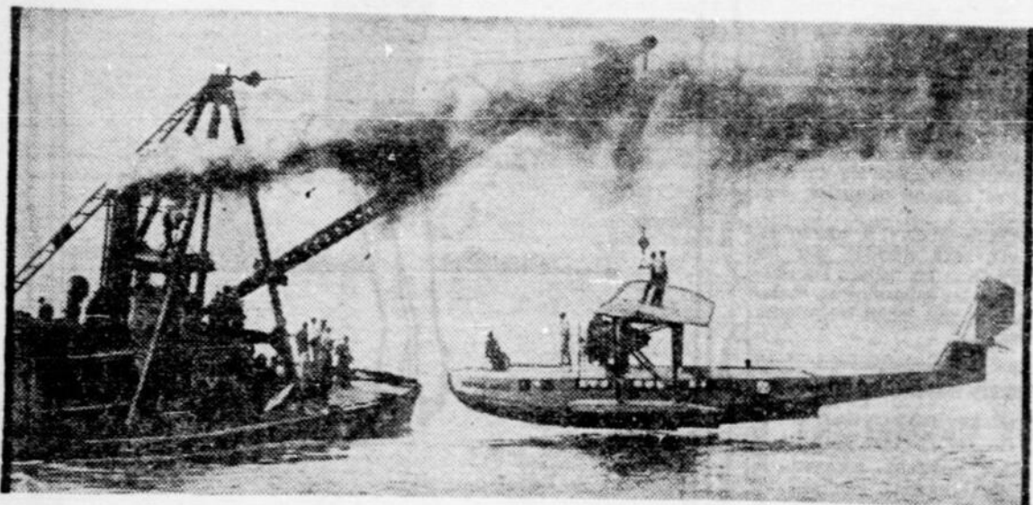
On assiste au lancement du plus gros hydravion américain dans la rivière Niagara. Cet hydravion, capable de transporter 32 passagers, a été construit à Buffalo et il est le premier d'une flottille de douze hydravions semblables qui seront affectés au service commercial entre New-York et Rio-de-Janeiro. D'autres iront jusqu'à Buenos-Ayres. Cet hydravion a une envergure de cent pieds et pèse 9,000 livres. Il coûte $100,000. On sait que le plus gros hydravion du monde est le "DO-X", fabriqué en Allemagne.
