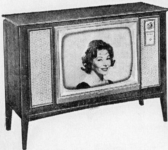
Le RANDALL • Modèle K2756R Console "Lo-Boy" Style Danois Moderne en Noyer et bois dur massif. Syntonisateur. 2 gros haut-parleurs de 9". Circuit automatique. Contrôle dynamique. Lampe-écran "Super Sunshine"®. Dimensions : hauteur 32", largeur 42-11/16", profondeur 16 1/8".
