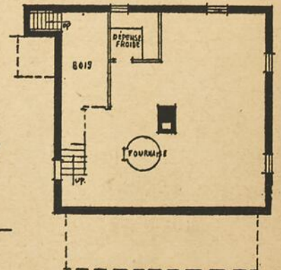
SOUS-SOL
