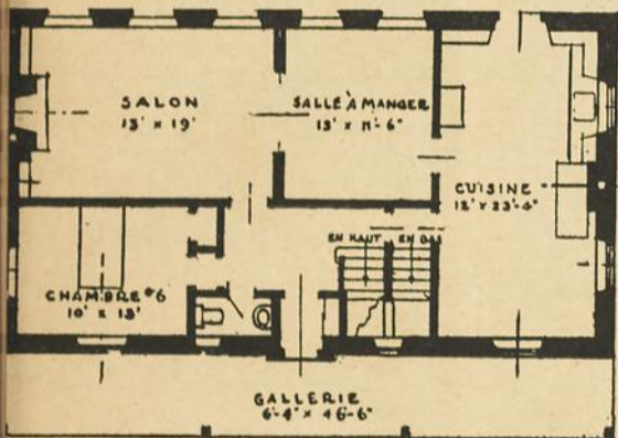
REZ-DE-CHAUSSÉE
