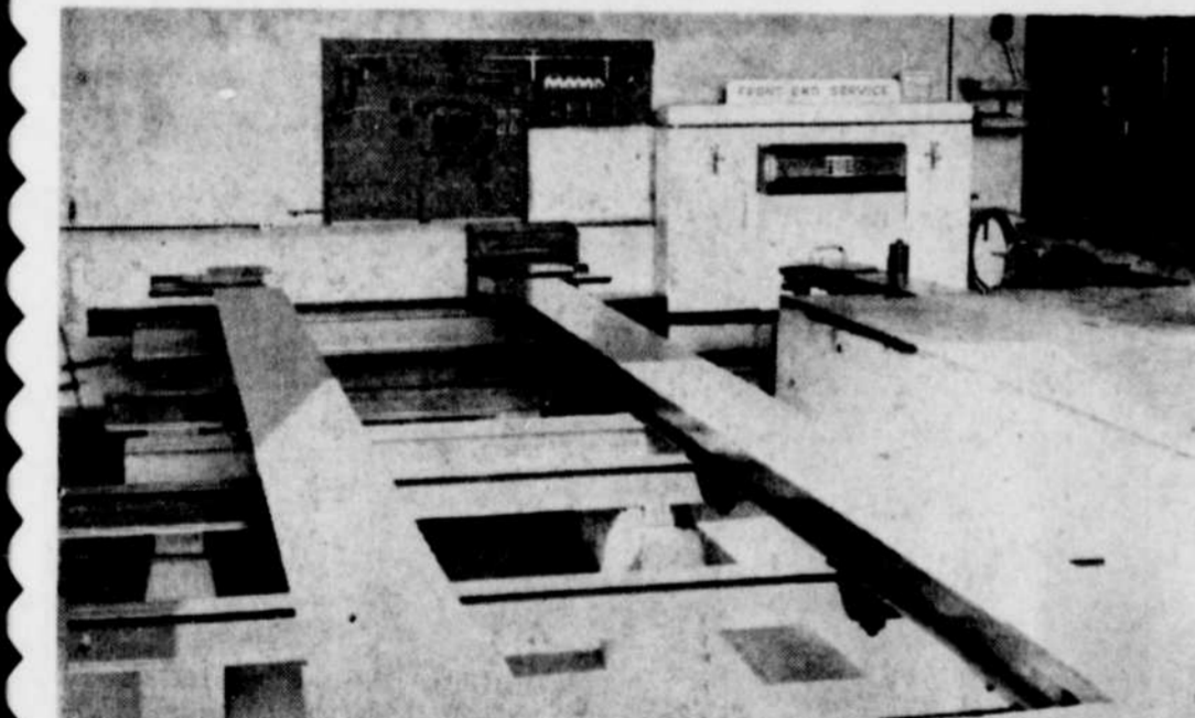
La photo ci-haut vous fait voir nos nouvelles machines "BEAR" pour le redressement des châssis et des essieux, ainsi que pour l'alignement et le balancement des roues. Ces machines donnent un rendement impeccable sur toute voiture, ainsi que sur camions, (jusqu'à 10 tonnes).
