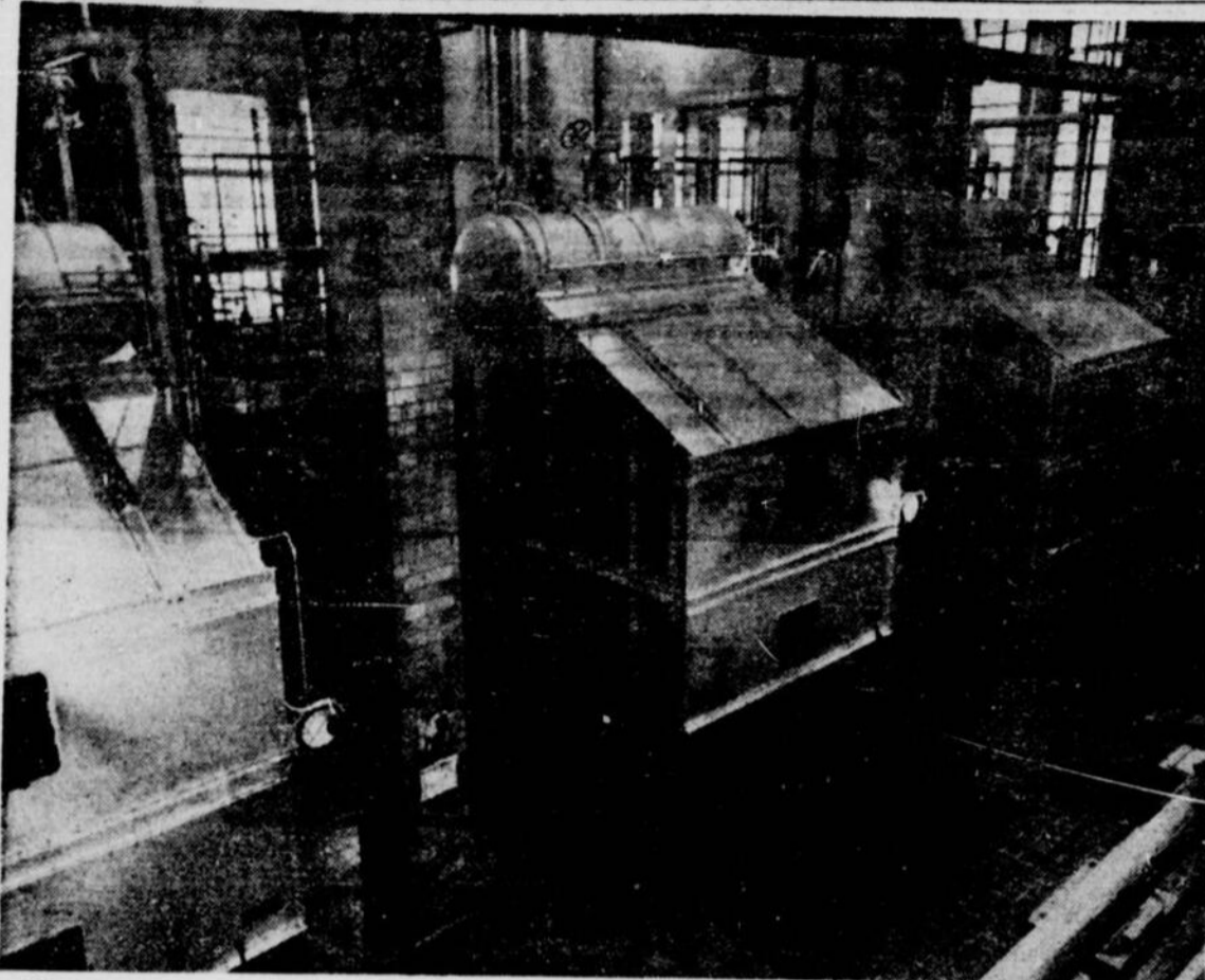
CHAUDIÈRES A VAPEUR. — On voit ici les trois chaudières à vapeur de la chaufferie du nouvel Hôpital Sainte-Justine. Ces immenses chaudières, d'une hauteur de 20 pieds et d'une capacité individuelle de 1,000 chevaux-vapeur, fonctionnent à l'huile, mais peuvent être aussi adaptées pour le chauffage au charbon. Elles fournissent la chaleur sur une superficie totale de 1,400,000 pieds carrés et procurent aussi la vapeur et l'eau chaude domestique pour tous les services: buanderie, cuisine, ventilation, air climatisé et stérilisation. Deux chaudières seulement seront habituellement en opération. La troisième est une chaudière supplémentaire, pour parer à toute éventualité, car un hôpital ne doit jamais manquer de chauffage.
