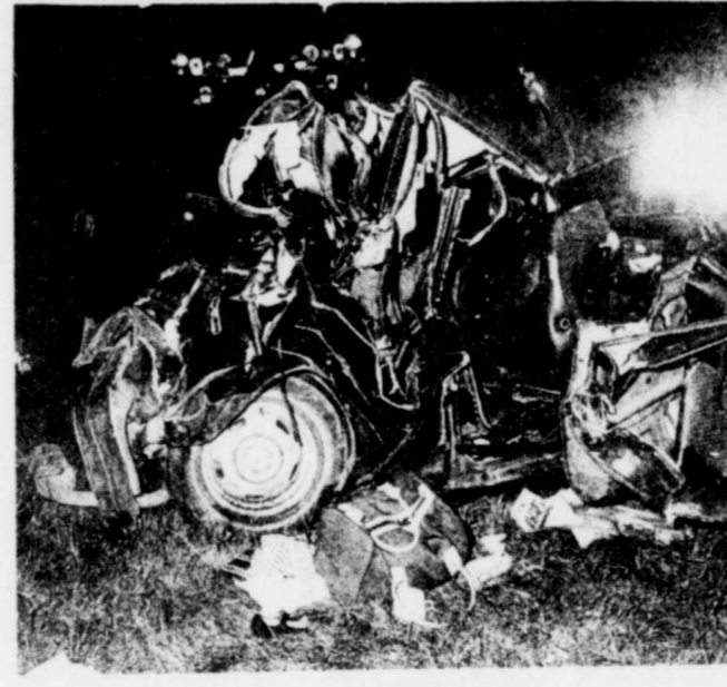
Le pare-choc du 4x4 était plus élevé que celui de la Volvo (collision par l'arrière, à 65 km/h).
