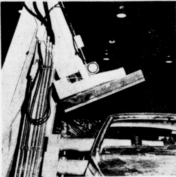
Un piston s'apprête à emboutir le toit d'une voiture: simulation d'un capotage.
