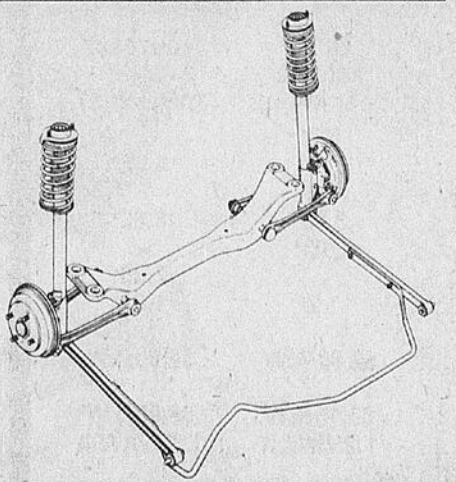
Suspension arrière entièrement indépendante, qui se traduit par une excellente maniabilité.
