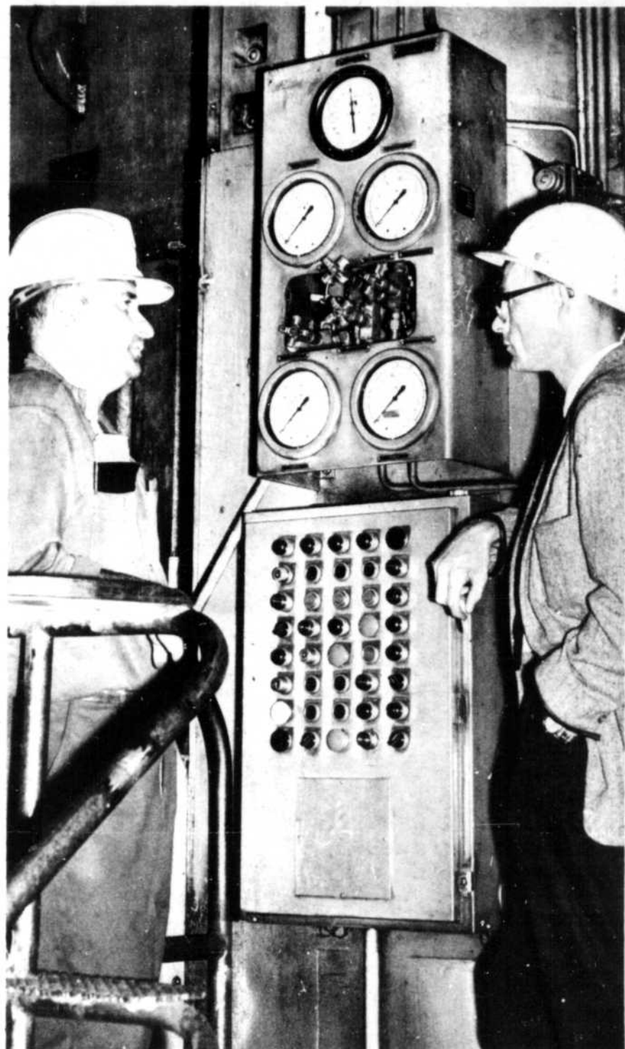
UNE PRESSE HYDRAULIQUE DE 60 PIEDS DE HAUTEUR — Même si la photo ne montre que les cadrans indicateurs de la presse hydraulique que l'on a installée à l'usine des électrodes de l'Alcan d'Arvida, le lecteur peut facilement s'imaginer la grosseur d'une presse de 60 pieds de hauteur. A gauche, M. Louis-Guérin Pelletier, contremaître de quart de la presse H.P.M., s'entretient avec le surveillant du contrôle de la qualité de l'usine des électrodes, M. H. Topham.
