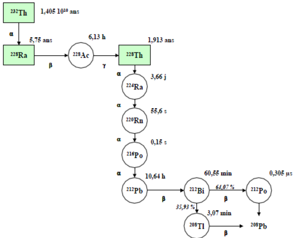
Figure 1 – Chaîne de désintégration du thorium.
