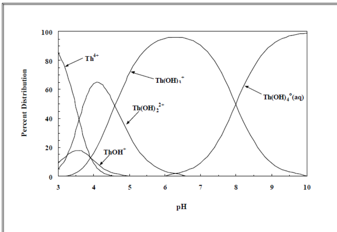
Figure 2 - Distribution des espèces de thorium hydrolytiques en fonction du pH. La répartition des espèces est basée sur une concentration de 1 µg/l de thorium total dissous dans de l'eau pure (par exemple, absence de ligands complexants autres que OH - ) et sur les données thermodynamiques de Langmuir et Herman (1980). Figure tirée de EPA (1999).
