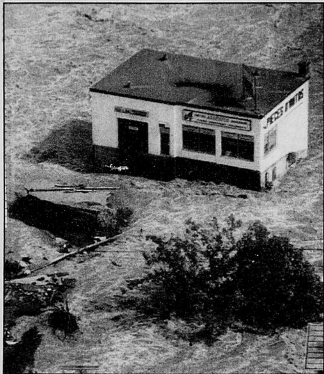
On peut avoir une très bonne idée de la force du courant quand on s'aperçoit que les fondations de ce garage de Chicoutimi ont été complètement déterrées par l'érosion.
