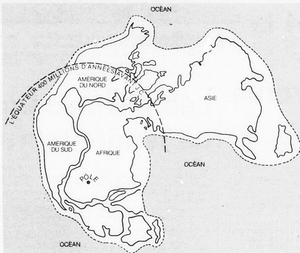
Comment ces roches pétrolifères ont-elles été formées dans les déserts glacés de notre Grand Nord? Selon les géologues, les continents se sont lentement déplacés si bien qu'il y a environ 400 millions d'années, les îles de l'Arctique se trouvaient proches de l'équateur. La chaleur et la pression créées par ce mouvement ont transformé les sédiments du fond de la mer en pétrole brut. Mais il faut beaucoup d'expérience et un rien d'intuition pour en dénicher la présence.
