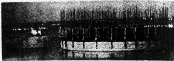
Mise en place d'un premier caisson au petit matin sur le fleuve Saint-Laurent.
