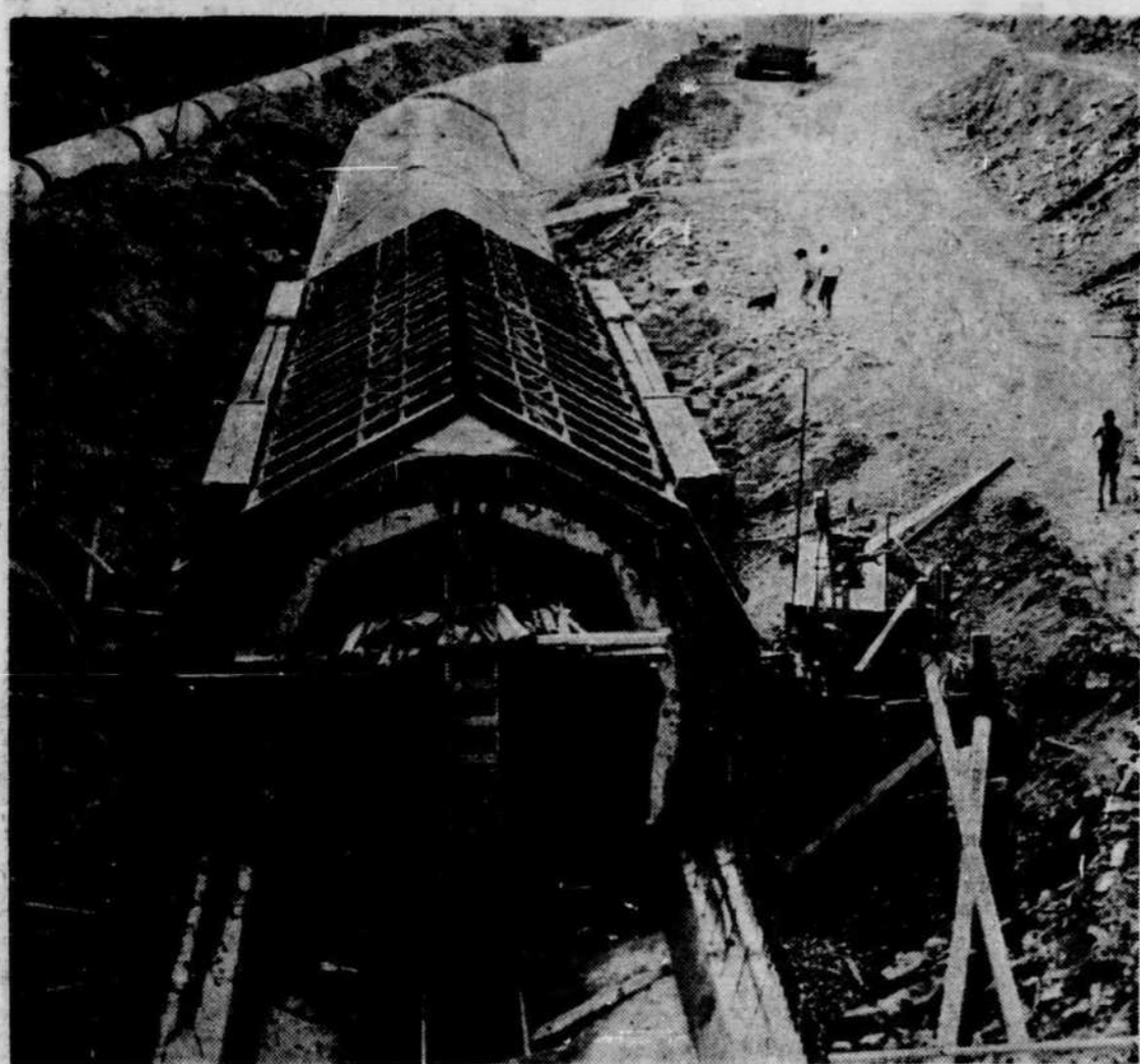
LA CONSTRUCTION D'UNE IMMENSE CONDUITE reliant les limites de la ville de Charlesbourg à la rivière Saint-Charles, sera bientôt complétée. Cet énorme tuyau de 12 pieds à l'intérieur, mesure pas moins de 6,000 pieds. Présentement, les ouvriers de la firme J.-A. Auclair procèdent aux travaux de finition de la dernière étape. Les dépenses pour cette phase finale, seraient évaluées à $215,000. La canalisation de la rivière Lairet, à partir de Charlesbourg jusqu'à la rivière Saint-Charles a coûté, disons-le, près de trois millions de dollars. Ce projet d'envergure comprendrait trois étapes. Sur la photo, nous pouvons voir une partie de la conduite, laquelle sera entièrement nivelée au niveau de la partie est de la berge la plus basse, rue Cadillac.
