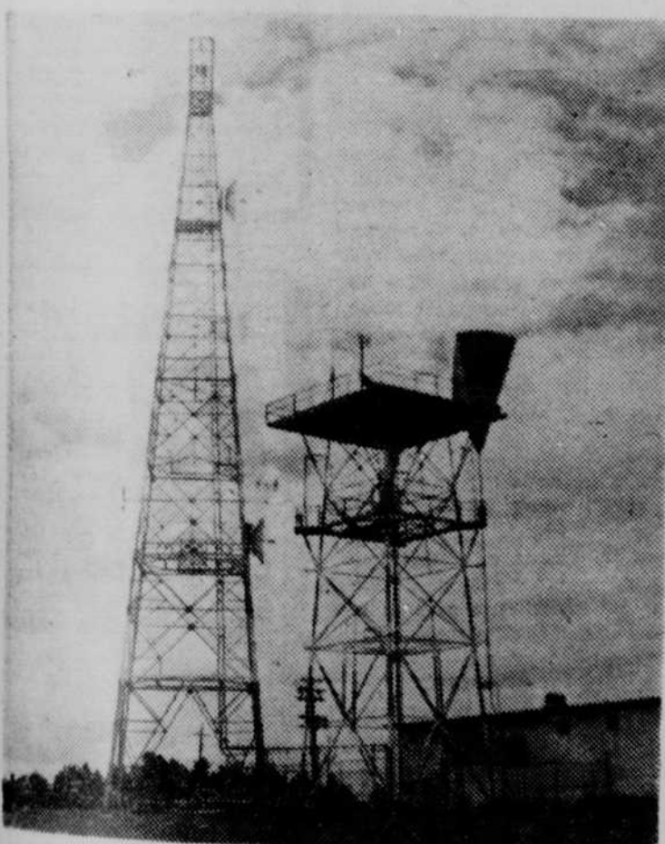
RIVIERE-DU-LOUP possède un système de communication des plus complets. Cette photo nous fait voir deux tours érigées par la Compagnie de Téléphone Bell du Canada. A gauche, une tour de relai du Réseau Trans-Canadien de Télévision et de Téléphone, et, à droite, une des trois tours (les deux autres s'élèvent sur la rive nord) du réseau de dispersion troposphérique qui élimine l'usage d'un câble sous-marin entre les deux rives.
