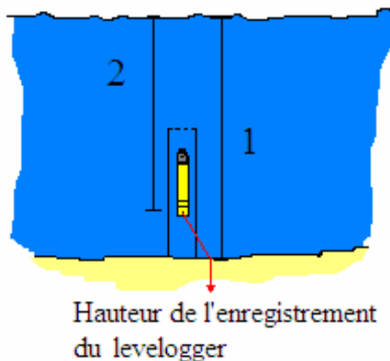
Figure 12 : Schéma illustrant les mesures faites avec le poids de sonde. (1) Hauteur d'eau du lac ; (2) Hauteur de l'enregistrement.
