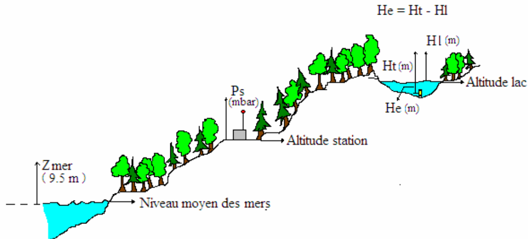
Figure 21 : Schéma illustrant la nécessité d'une compensation barométrique. Compensation barométrique
