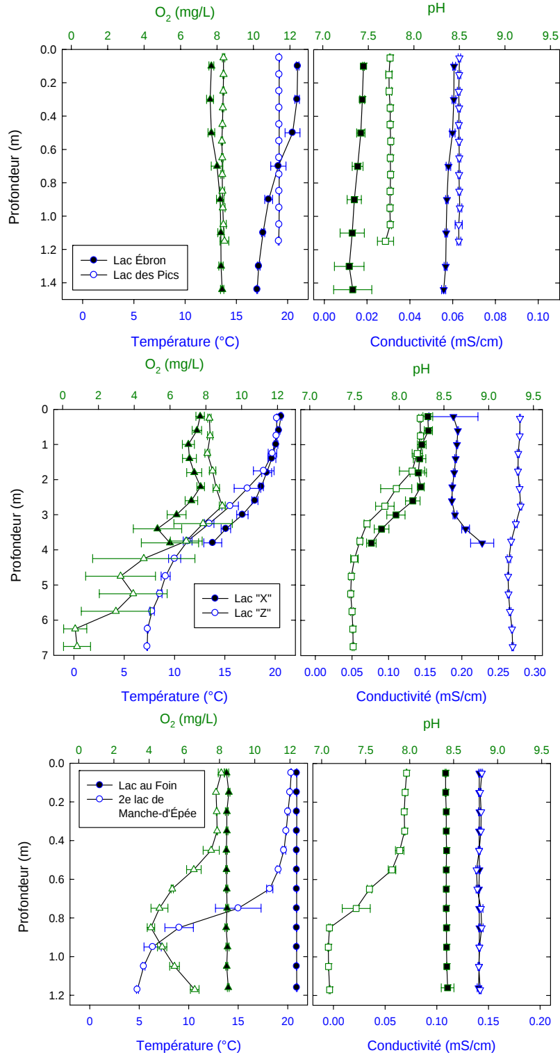
Figure 15 : Profils verticaux de quatre paramètres mesurés par sonde submersible dans chaque paire de lacs entre les 17 et 19 juillet 2007 (●○ : Température ; ▲△ : O 2 dissous ; ■□ : pH ; ▼▽ : Conductivité)
