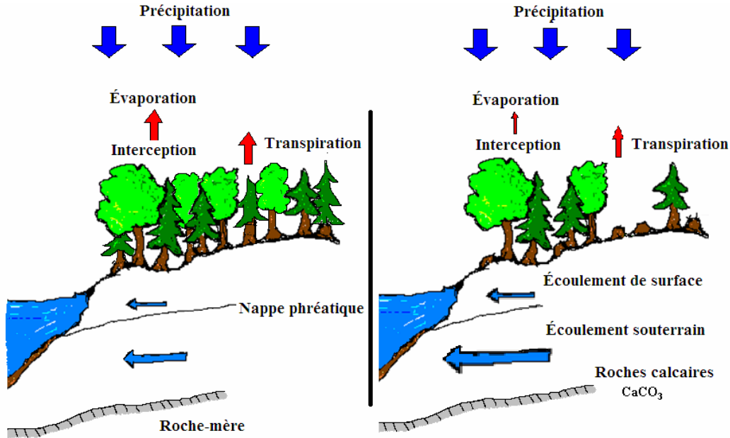
Figure 1 : Schéma simplifié de l'influence de la récolte forestière sur le bilan hydrologique
