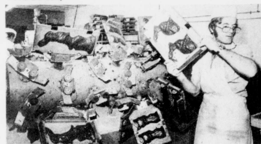
Après avoir refermé la plaque de bois qui comprend toujours les moules de plastique, on fixe le tout à ce cylindre rotatif. Celui-ci tournant dans le sens inverse de celui des moules, le chocolat se répand uniformément laissant le centre vide. (Photo Bernard Braut)
