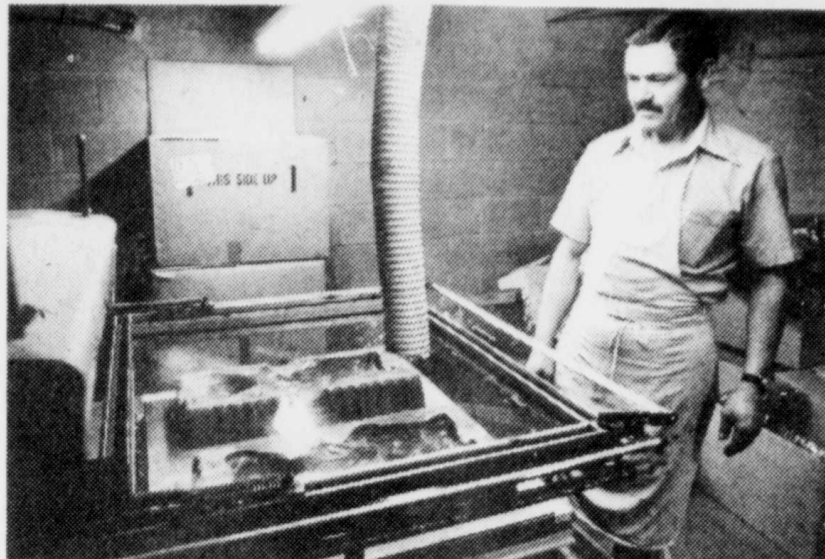
Au-dessus d'un premier moule de matière extra dure, une feuille de matière plastique est chauffée sous cette vitre; quand elle est ramollie au maximum, une sorte de presse arrive facilement à lui donner la forme du moule initial. (Photo Bernard Braut)
