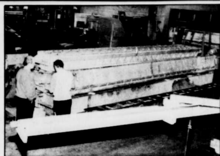
Les travailleurs de Laperrière et Verreault s'apprennent à modifier ces boîtes à succion afin de les adapter à la table de Fourdrinier pour la machine de l'usine de Port-Cartier.
