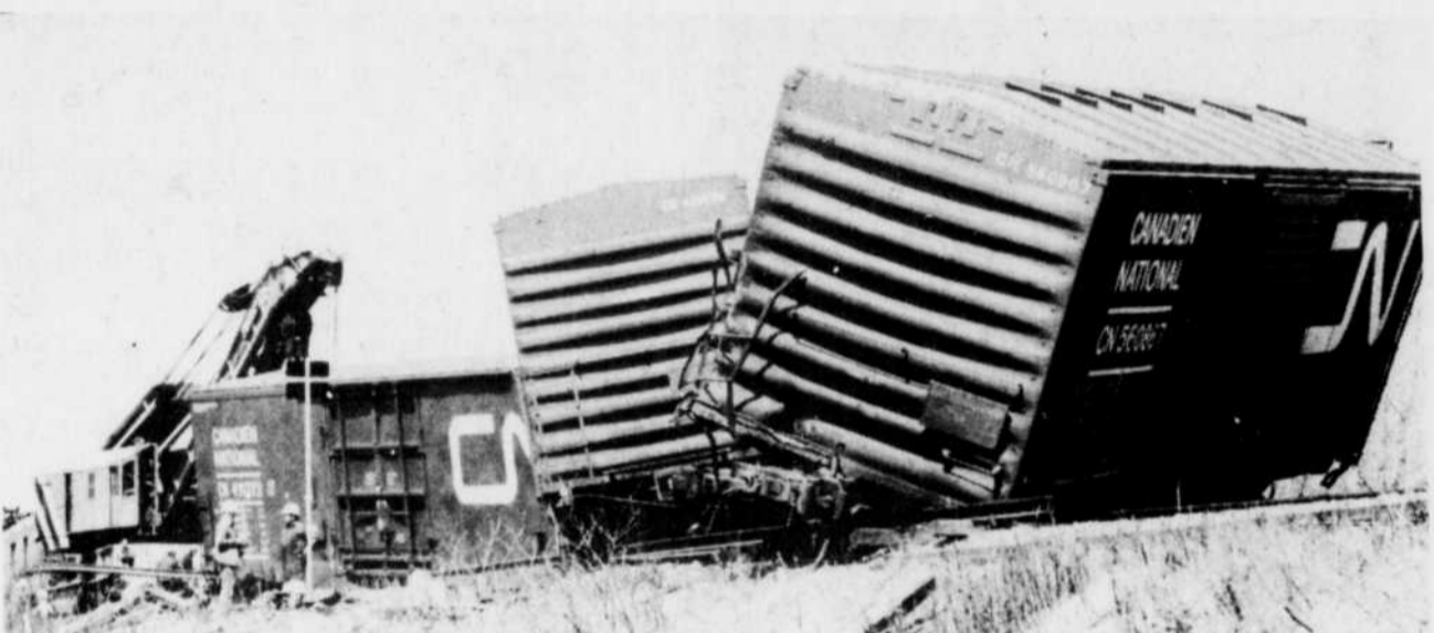
Une grue montée sur une plate-forme du Canadien national, grâce à des câbles d'acier très résistants, a prêté main forte au bélier mécanique pour ramener les wagons dans le droit chemin.
