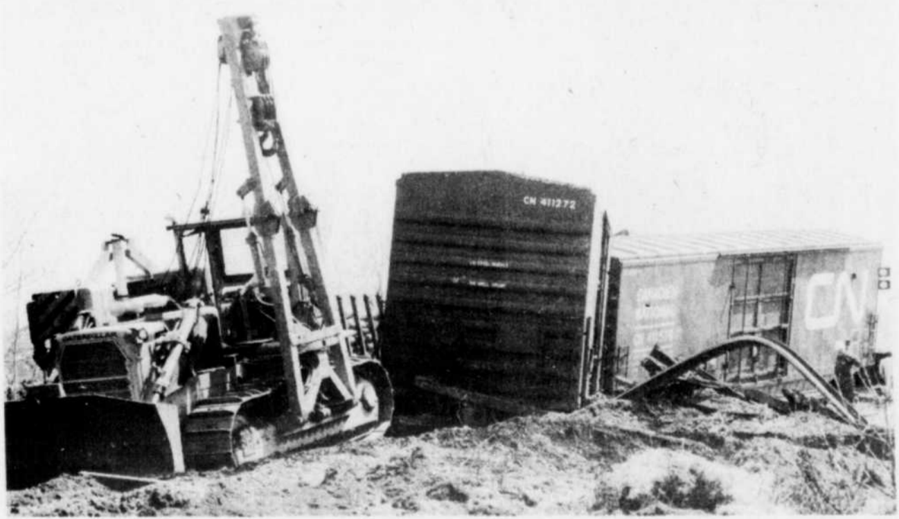
Grâce à un bélier mécanique pesant 85 tonnes et muni de deux contrepoids pesant chacun 13 tonnes, on a pu pousser et tirer les wagons qui pesaient environ 160 tonnes.
