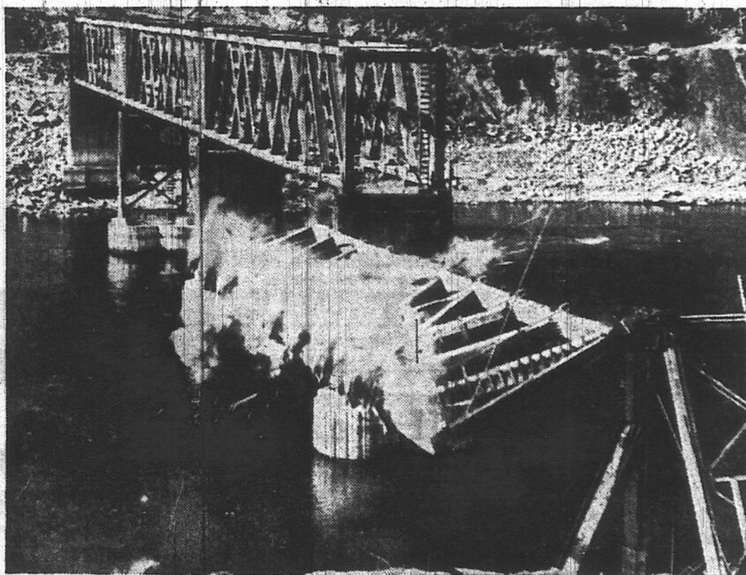
Ce pont en fer avait été érigé temporairement pendant la construction du barrage Grand Coulee, à Washington. Les travaux étant terminés, on a simplement détruit le pont à la dynamite, comme on peut le voir dans la photo ci-dessus.
