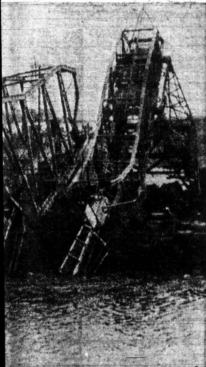
Il reste d'une grue géante de 60 tonnes, qui se préparait à démonter cette grue, qui était effondrée... Elle n'en pouvait plus de vieillesse. (Fac-similé United Press — "Montréal-Matin")
