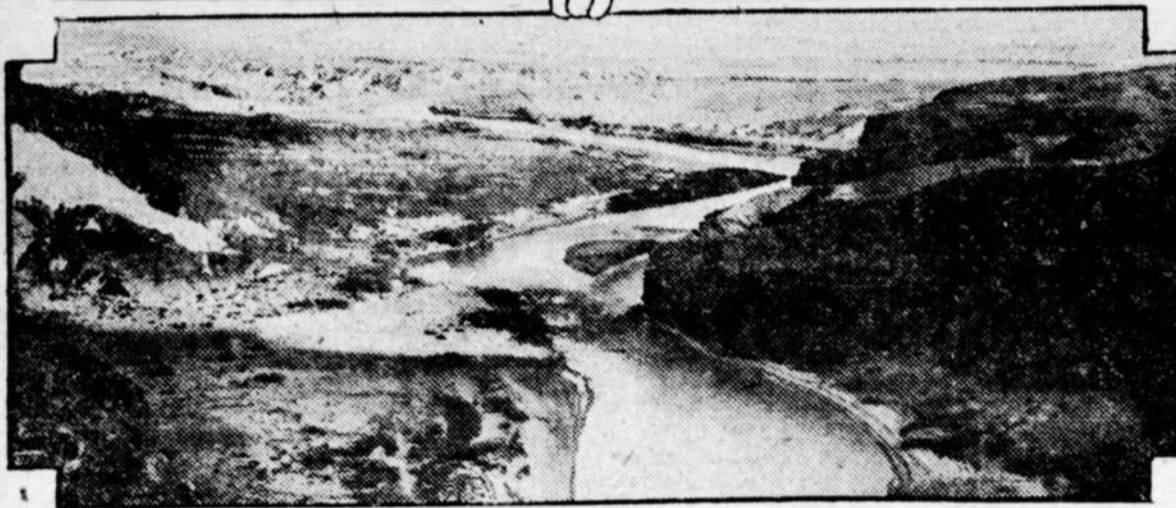
En haut: le Rhin à son arrivée dans le lac Constance. En bas: vue panoramique indiquant la vallée du Rhin où se poursuit un lent mais gigantesque travail d'usure.
