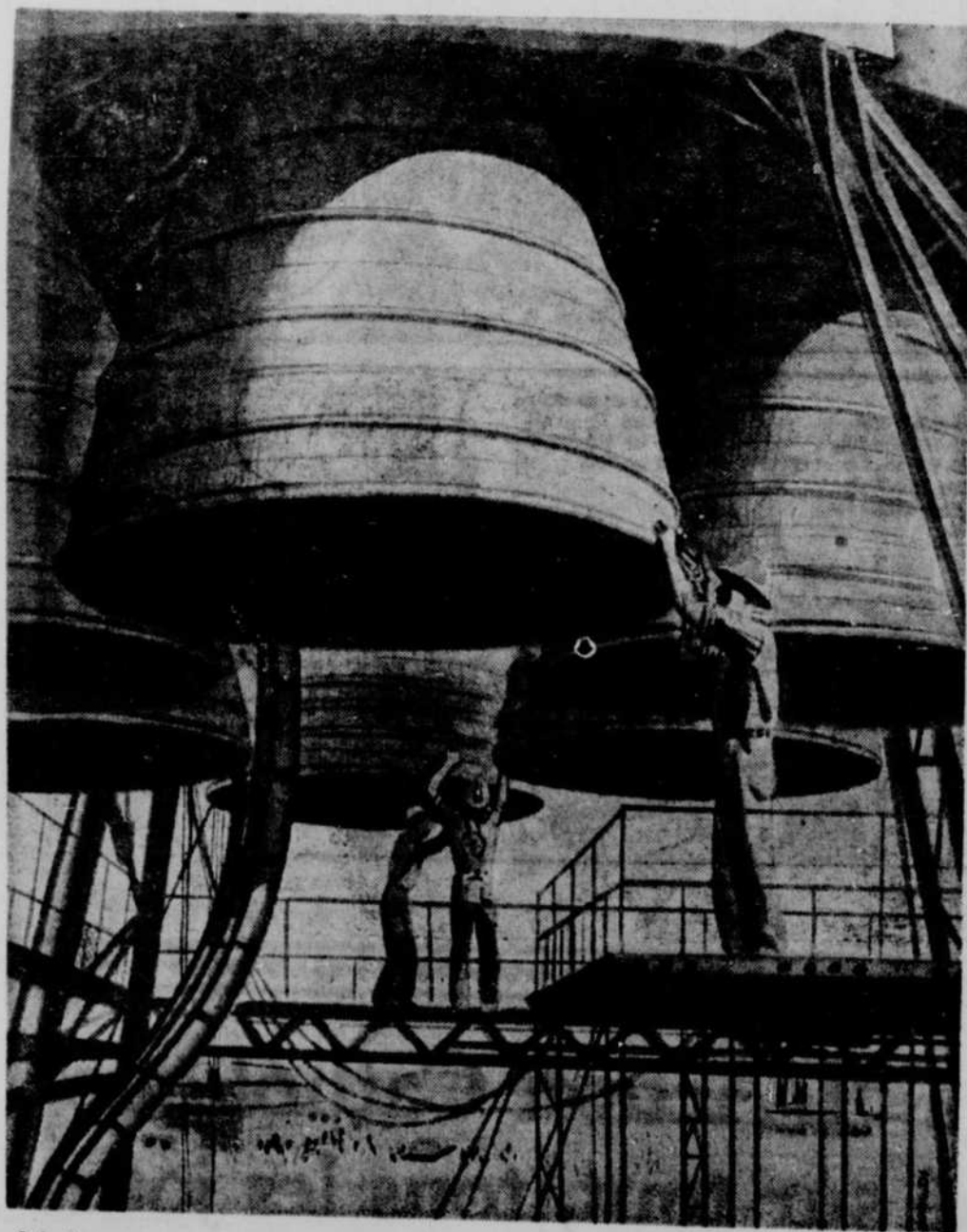
Une fois les moteurs de la Nova assemblée en groupe de six, l'on peut se rendre compte des possibilités de ce système.
