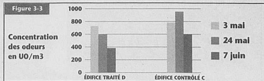
Figure 3-3, Évolution des concentrations d'odeurs aux sorties des ventilateurs des deux bâtiments.
