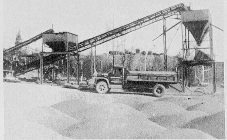
Machineries pour Graviers, Sables et opérations de ciments, installation électrique de 550 Volts. ST-GEORGES JERSEY-MILLS, Tél. 228-3111.
