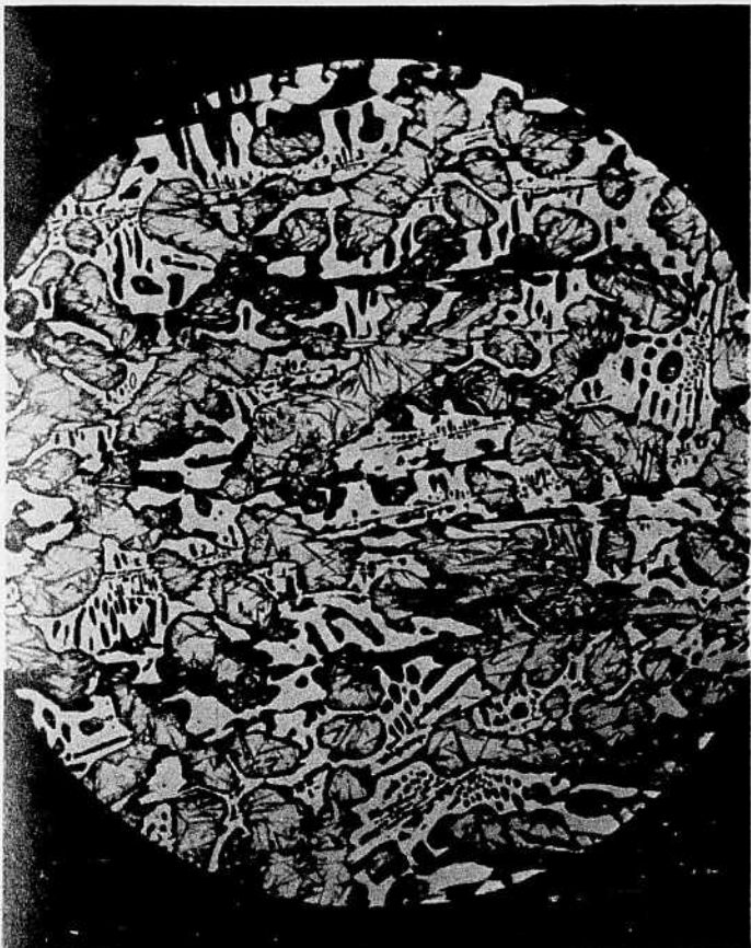
Voilà ce que le microscope électronique révèle à ceux qui regardent une particule de métal! En étudiant cet alliage de nickel, on en a fixé les limites de résistance et on a ainsi obtenu des renseignements supplémentaires qui ont permis ensuite la préparation d'un meilleur alliage.
