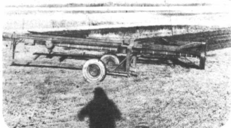
POMPE A FUMIER LIQUIDE
