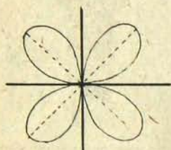
UNE ROSE DE GRANDI (x^2 + y^2)^3 = 4a^2 x^2 y^2
