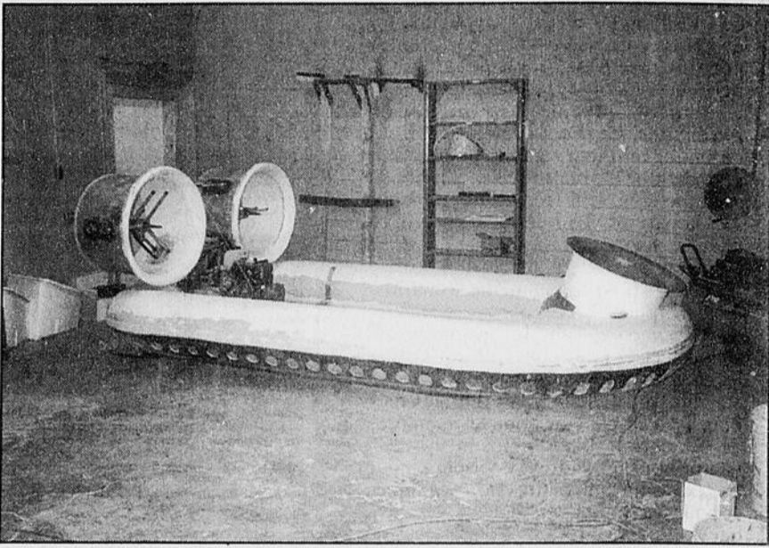
Une équipe de 13 étudiants de Sherbrooke et de Montréal a créé le Triton, un aéroglesseur qui sera exposé aujourd'hui au Pavillon central de l'Université de Sherbrooke.
