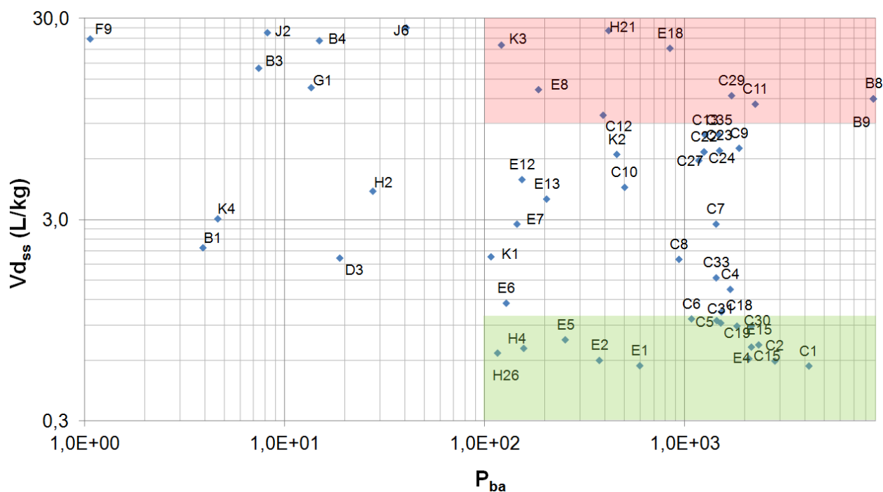
Figure 2 Présentation graphique des propriétés pharmacocinétiques ( Vd_{ss} et P_{ba} ) des 55 COVM retenus au niv. 4 (voir Tableaux 4 et 5 pour les codes assignés aux COVM).
