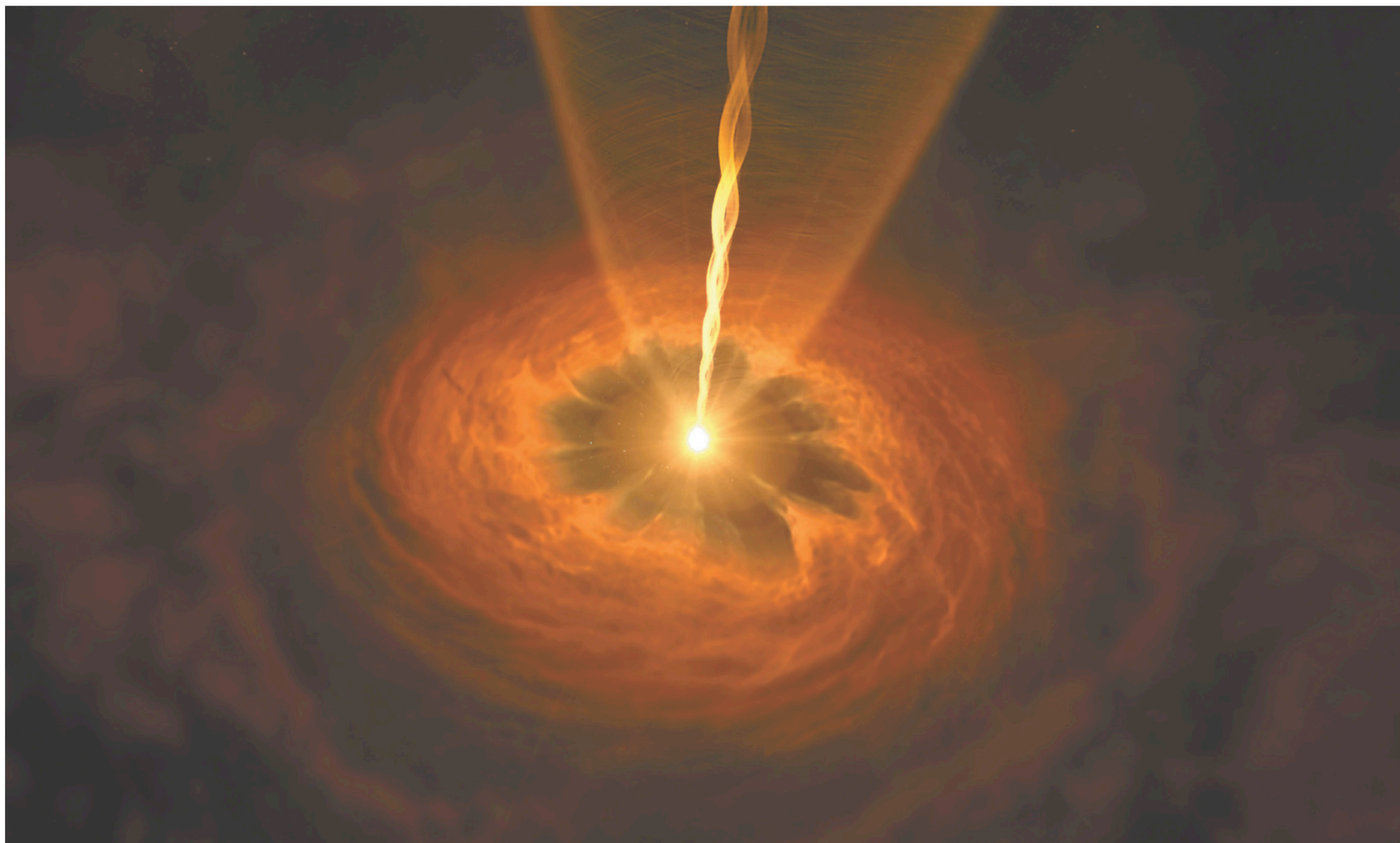
La formation de notre système solaire
