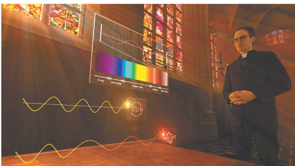
Le prêtre et astrophysicien belge Georges Lemaître constate que les spectres lumineux des nébuleuses qu'il observe sont décalés vers le rouge. Il comprend ainsi que l'Univers est en expansion.
