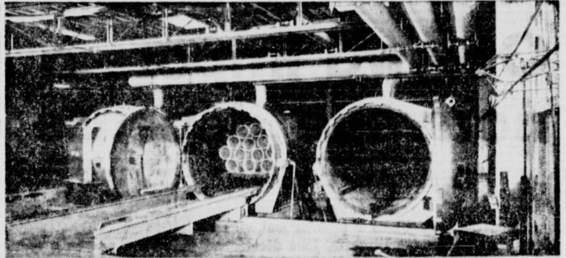
L'ATELIER AUTOCLAVE — Trois autoclaves, mesurant chacun plus de 100 pieds de longueur et 7 pieds de diamètre, font subir au tuyau définitivement ouvré, le procédé final de traitement à la vapeur. A noter que l'autoclave No 2 est rempli de tuyaux à pression "Turnall" de 8".
