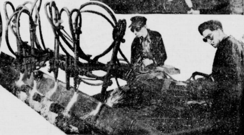
(Adroite) LA FABRICATION DES OBUS est très active dans les ateliers de CANCAR. On voit ici deux ouvriers préposés à ce travail. (Ci-dessous) LES DOUILLES D'OBUS sont faites de feuilles d'acier qui sont ainsi coupées en longueur à l'aide d'un outillage perfectionné qui permet d'effectuer ce travail avec rapidité et précision.
