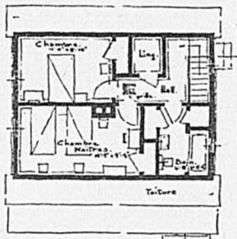
PLAN D'ÉTAGE
