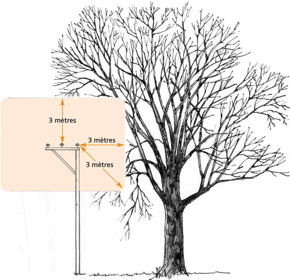
Illustration n° 52 Travaux à proximité d'un réseau électrique aérien
