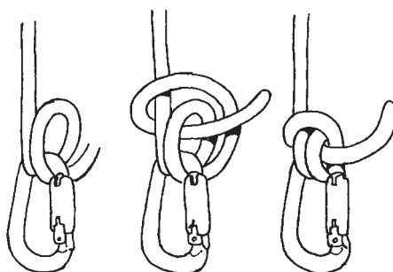
Illustration n° 5 Nœud d'ancre
