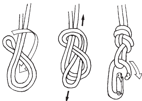
Illustration n° 4 Nœud en huit double
