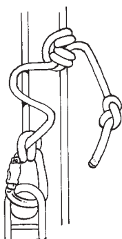
Illustration n° 15 Méthode traditionnelle
