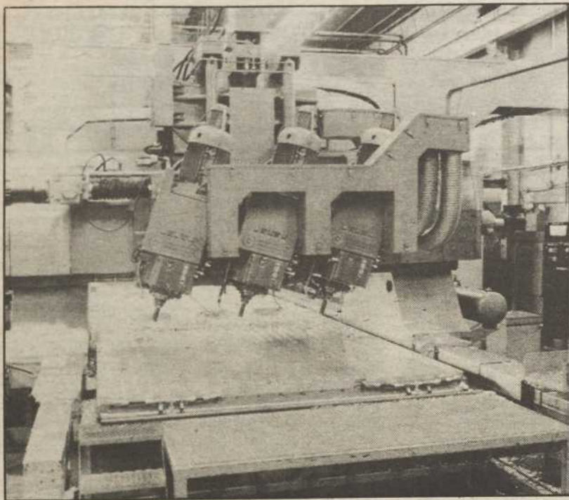
Cette fraiseuse à cinq axes est fabriquée par la firme française Machines-Outils Henri Liné de Granby.
