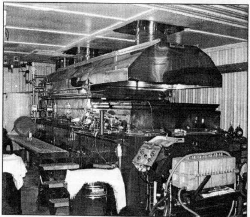
L'évaporateur Thunderbolt- la cadillac des évaporateurs à l'Érablière Turgeon-Gagnon
