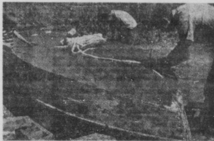
Fig. 1: Si vous devez poser du coton à calfater, prenez garde de ne pas en mettre trop, de peur de voir le bordé se disjoindre une fois renflé par l'eau!
