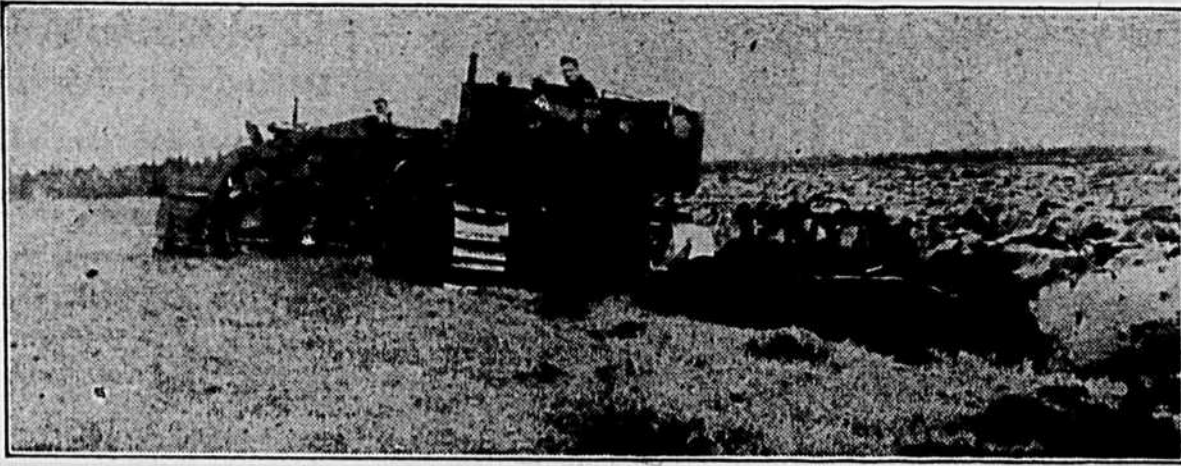
Les deux tracteurs que l'on voit ci-dessus, l'un de 65 et l'autre de 85 c.v., sont attelés à la charrue défonceuse utilisée par les cultivateurs du comté de Champlain pour amender les terres sablonneuses par l'apport de glaise extraite du sous-sol. (Voir en page 7 d'autres photos et l'article de M. Fleury). (Photo du Service provincial de Cine-Photographie)
