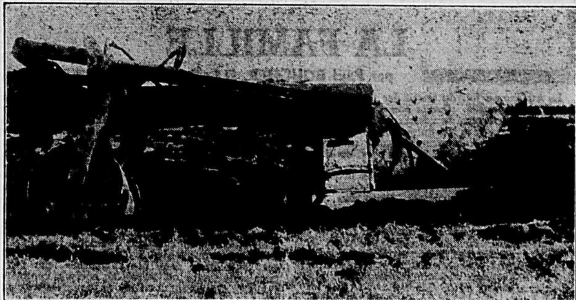
Vue de côté de la charrue défonceuse qui mesure 20 pieds de longueur. Propriété de l'outillage de ferme de Québec, cette charrue rend de grands services aux cultivateurs de St-Luc de Champlain. D'un poids de trois tonnes et demie, elle trace un sillon de 38 pouces de largeur. La profondeur est réglée à volonté (Photo du Service provincial de Ciné-Photographie)
