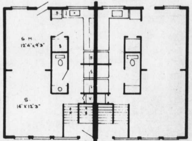
PLAN DE L'ETAGE 20 X 30'
