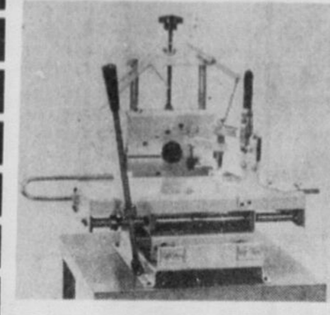
MORTAISEUSE-TENONNEUSE VERSATILE BERLIE
