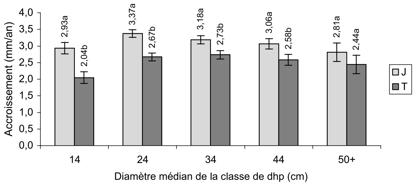
Figure 4. Accroissements annuels périodiques moyens en diamètre.
