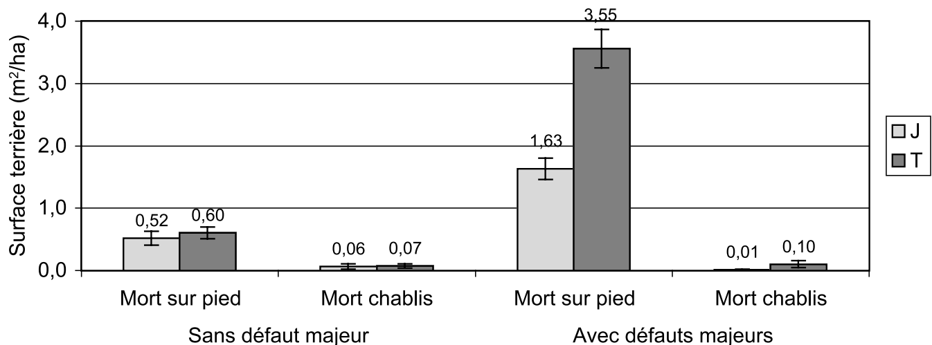
Figure 5. Répartition moyenne de la mortalité en surface terrière.
