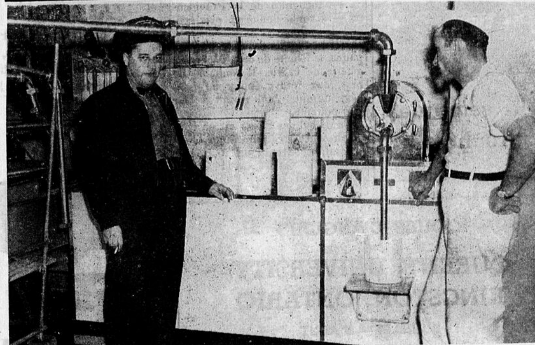
Sur la première photo, on peut remarquer une partie de la machinerie utilisée à La Laiterie de Louiseville pour la pasteurisation et l'homogénéisation du lait et de la crème ainsi que pour la fabrication de la crème glacée.
