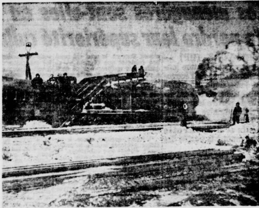
(Photos Canadian Pacifique) courroie sans fin. La neige est ainsi déversée dans une chaudière dont l'eau est réchauffée par la vapeur venant de la locomotive. La neige fondue est dirigée vers une bouche d'égout ou vers tout autre endroit propre à en faciliter l'écoulement.
