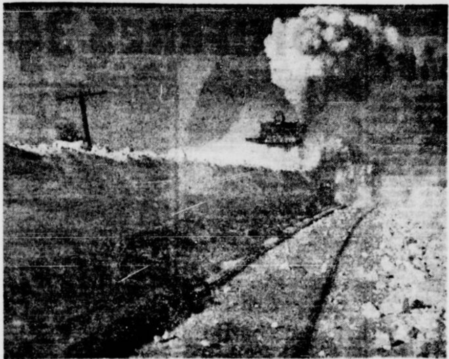
Ces photos, prises à la gare de triage Sortin du Canadien Pacifique, à Montréal-Ouest, font voir, à gauche, une charrue, et, à droite, une machine à fondre la neige en pleine opération. La charrue nettoie la voie tandis que la fondeuse recueille la neige au moyen d'un convoyeur pourvu d'une
