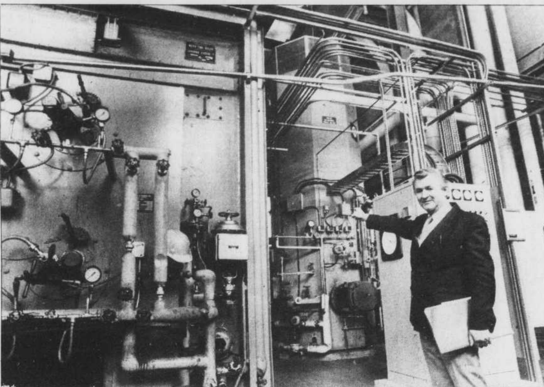
La partie droite de la photo montre la nouvelle génératrice à vapeur de l'hôpital Notre-Dame, qui permet à elle seule d'obtenir des économies annuelles de $328,000. À gauche, on aperçoit une génératrice traditionnelle, qui fonctionne à l'huile lourde avec un coût plus élevé, tout en laissant des odeurs et une pollution que le nouveau système ignore. M. Jacques Charbonneau, conseiller en communications de l'hôpital donne des explications.
