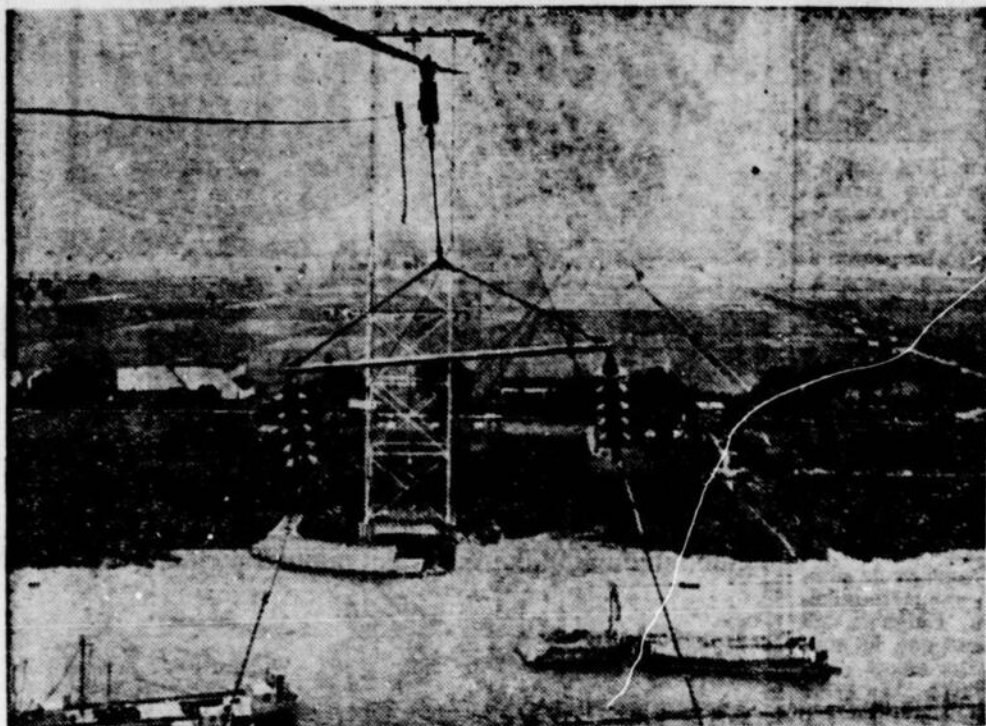
En cette photo, on aperçoit le gigantesque pylône sur la rive nord du fleuve, à proximité de la banlieue de Trois-Rivières. On peut voir le gros câble porteur auquel est fixée l'attache à ressort soutenant les isolateurs et les deux câbles électriques à haute tension, à 200 pieds au-dessus de l'eau.
