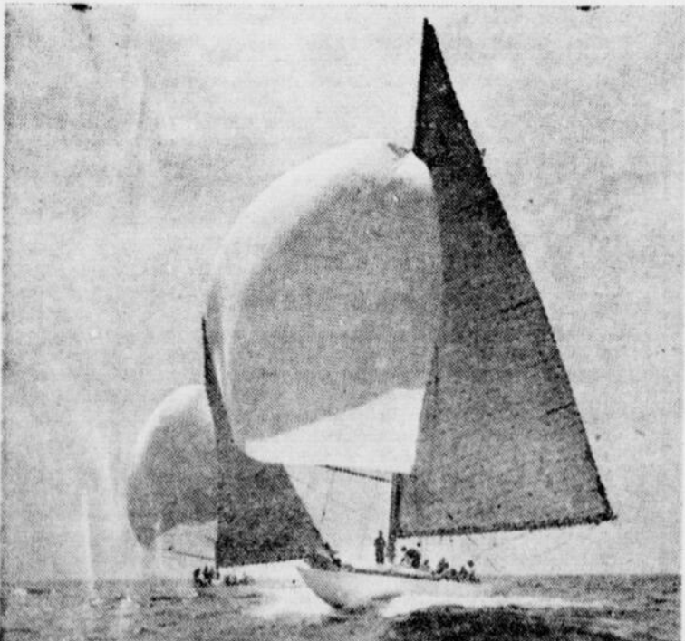
Fig 2: VOILES EN CISEAUX, au vent arrière. La poussée reçue par la grand-voile est contrebalancée par celle du spinnaker. (Photo Yachting)
