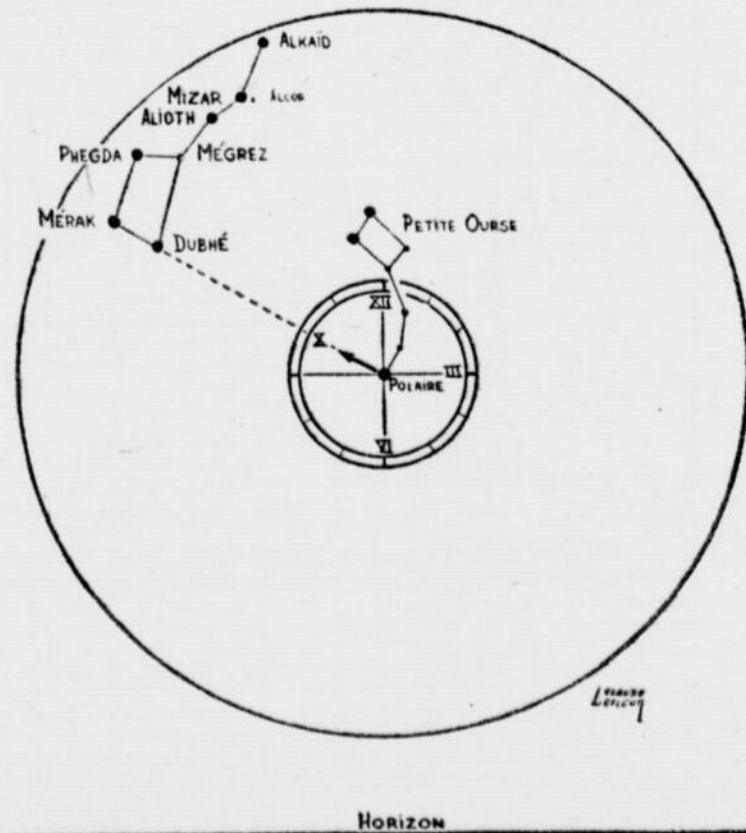
C'est la Grande Ourse vers 9 heures au début de juillet. La direction de la petite aiguille du cadran est celle de Merak-Dubhé.
