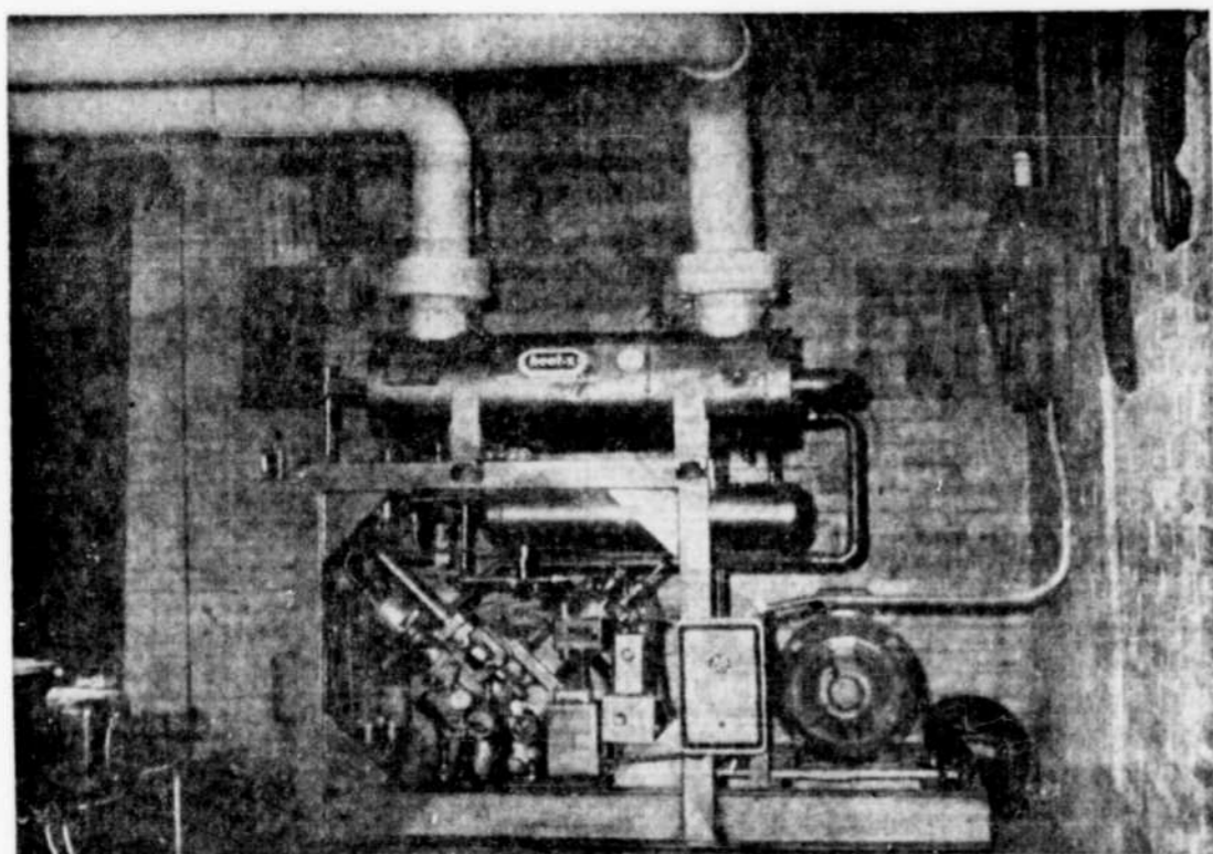
Voici l'installation du refroidisseur d'eau "HEAT-X" Frigidaire de l'édifice du Sherbrooke Trust
