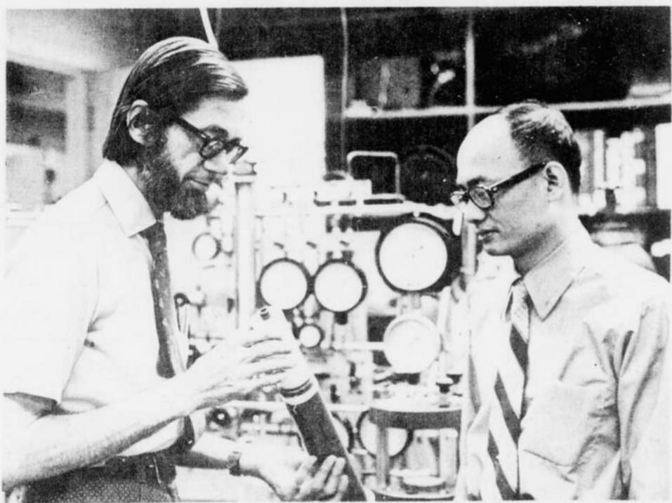
L'EXTRACTION DE L'HELIUM — MM. H.W. Habgood (à gauche) et C.Y. Pan, du Conseil de recherches de l'Alberta, examinant une membrane entourant un tuyau. Quand ce tuyau est placé dans une pipeline de gaz naturel, l'hélium passe à travers la membrane et sort par le tuyau central. On espère que ce procédé rendra l'extraction de l'hélium plus économique.
